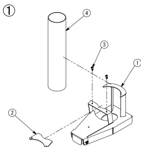
部品図
