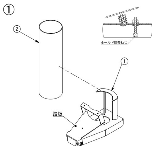
部品図
