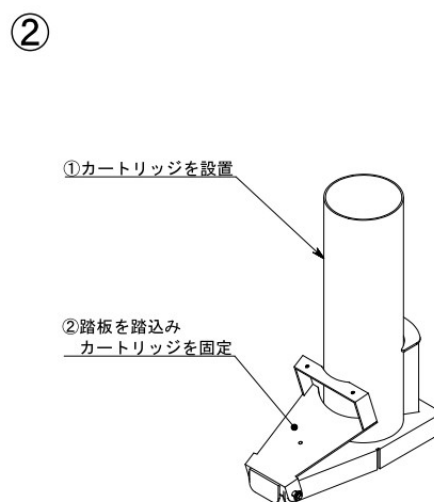
組立図
