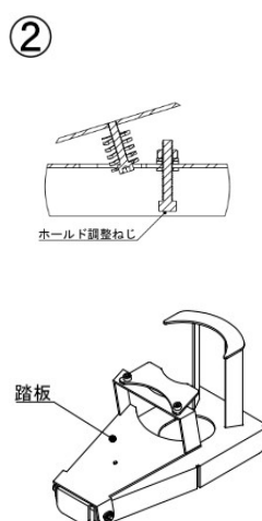
組立図
